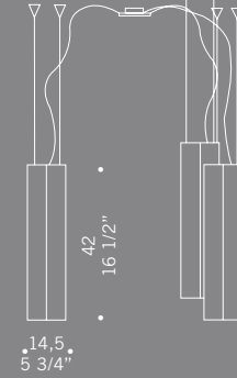
CARRÈ S3GD 3x70W E27 alogeno chiara clear halogen 3x26W E27 fluorescente fluorescent cavo elettrico 200 cm cables lenght 200 cm
