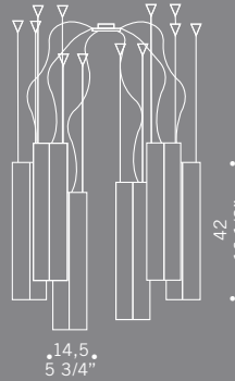
CARRÈ S6GD 6x70W E27 alogeno chiara clear halogen 6x26W E27 fluorescente fluorescent cavo elettrico 200 cm cables lenght 200 cm
